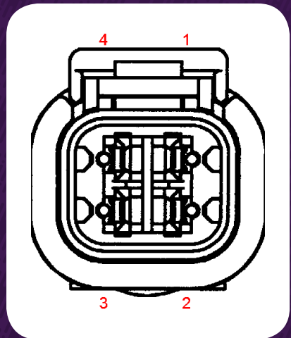
Deutsch 4-Way Connector Diagram
